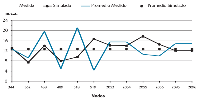
Figura 11. Curva comparativa de presiones. Sector Este.
