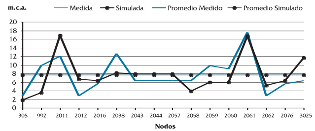
Figura 9. Curva comparativa de presiones. Sector Sur.
